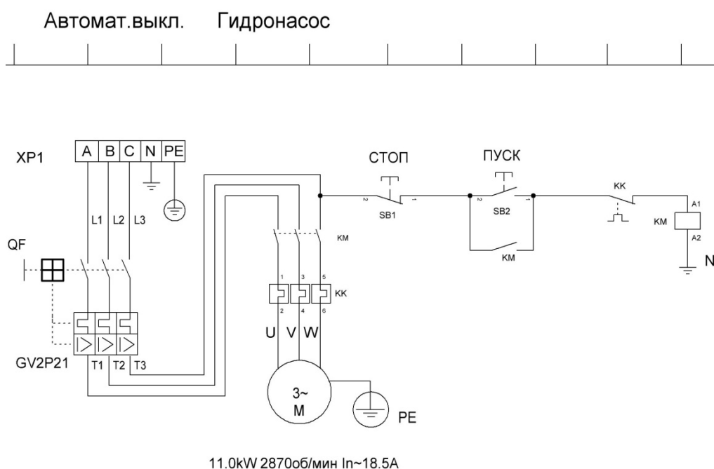
Рис. 2. Схема электрическая принципиальная 36Г272М1
