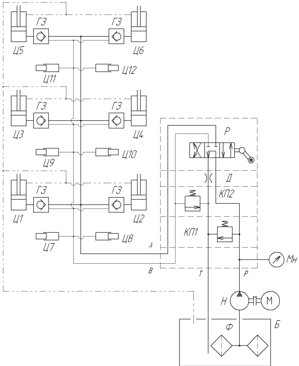
Рис. 3. Схема гидравлическая принципиальная 36Г272М1
